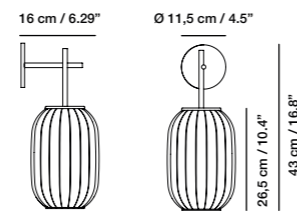
Difusor B
