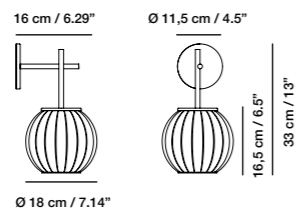
Difusor A
